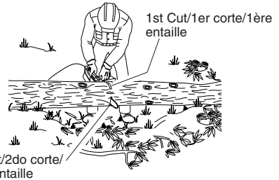
Figure 17 - Bucking Log When Log Is Supported On Both Ends Figura 17 - Trozado del tronco apoyado sobre ambos extremos Figure 17 - Tronçonnage d'une bille soutenue aux deux extrémités
